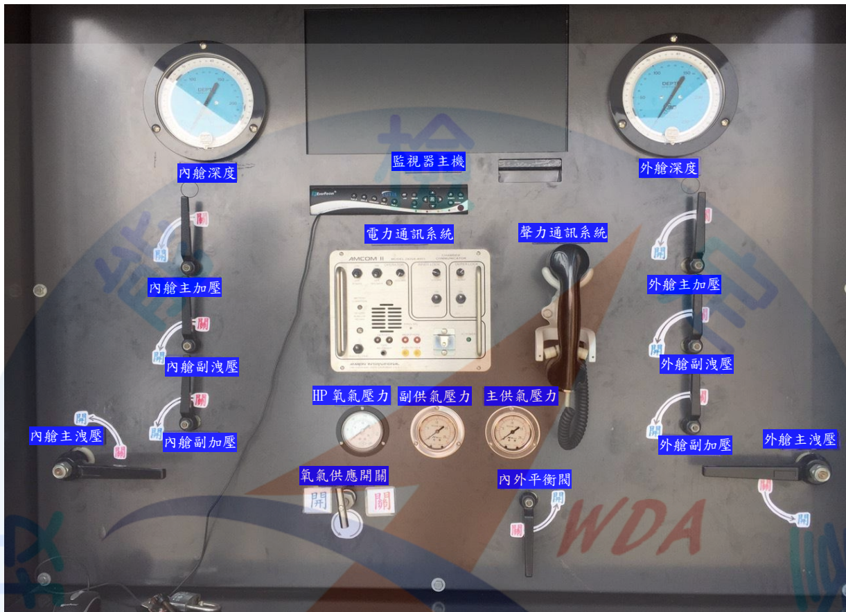
檢定用重壓櫃操控面板照片(範例)
